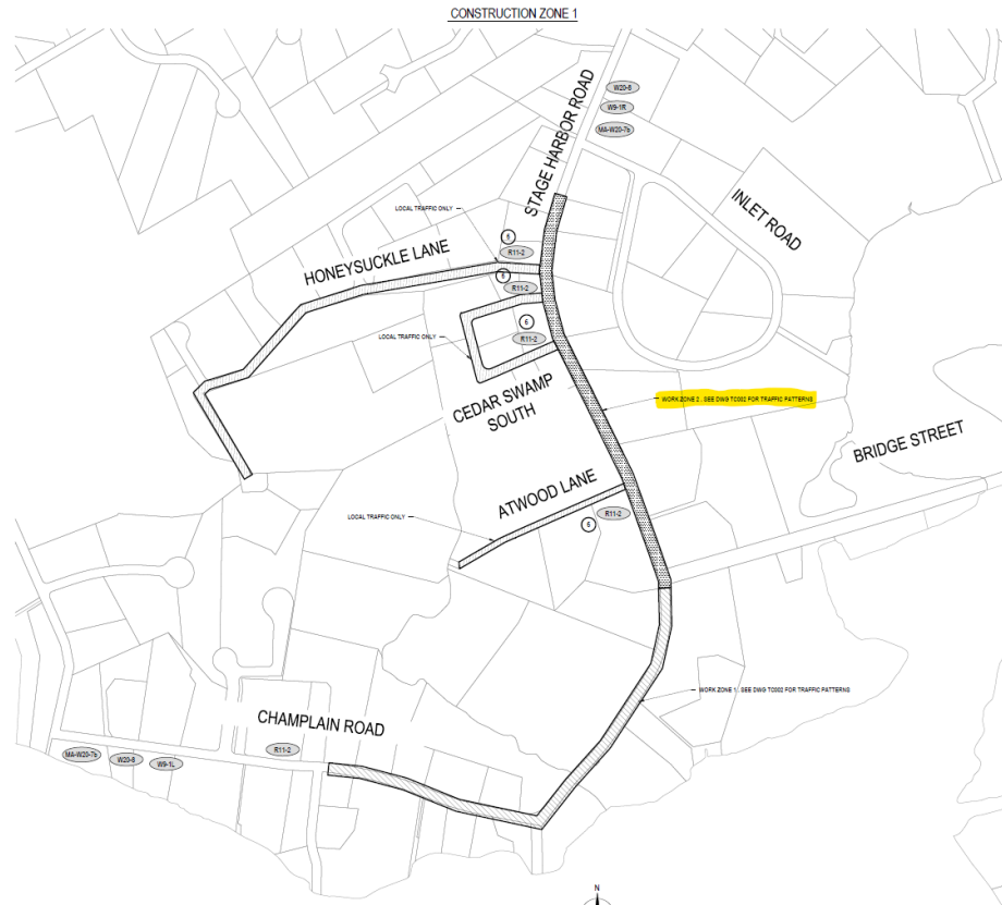
TRAFFIC CONTROL 1E - PLAN NTS
